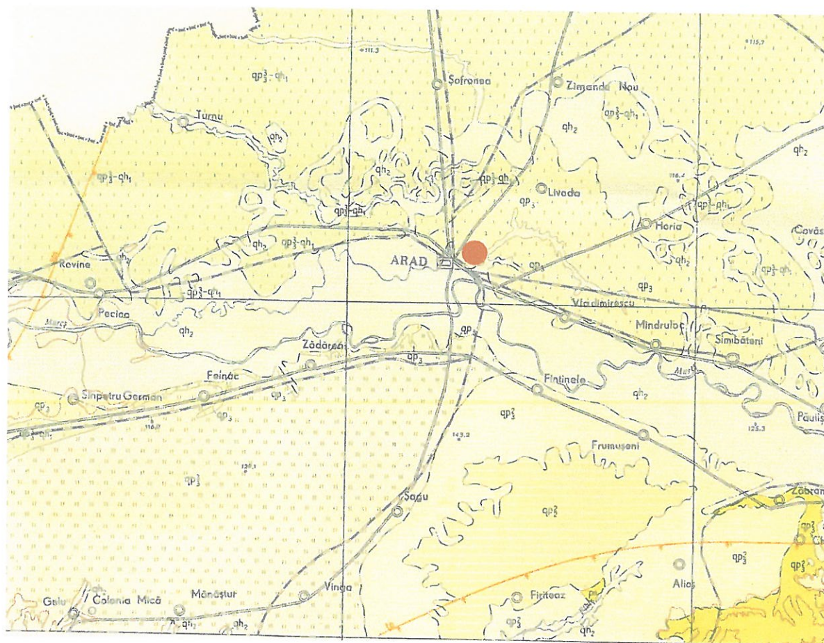
Imagina 1: Harta Geologică a României 1:200000, extras din Foaia 16 – Arad. ● zona de executie a lucrărilor geotehnice
